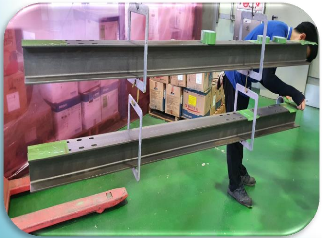
<< 에어작업 및 마스킹 >>
