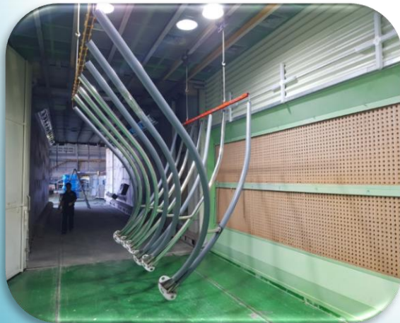
<< 수동식 OVEN 및 분체,액체 부스 >>
